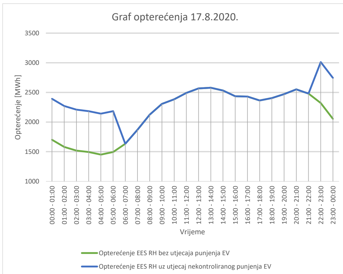
Slika 9. Usporedba opterećenja EES RH bez utjecaja i s utjecajem nekontroliranog punjenja EV
