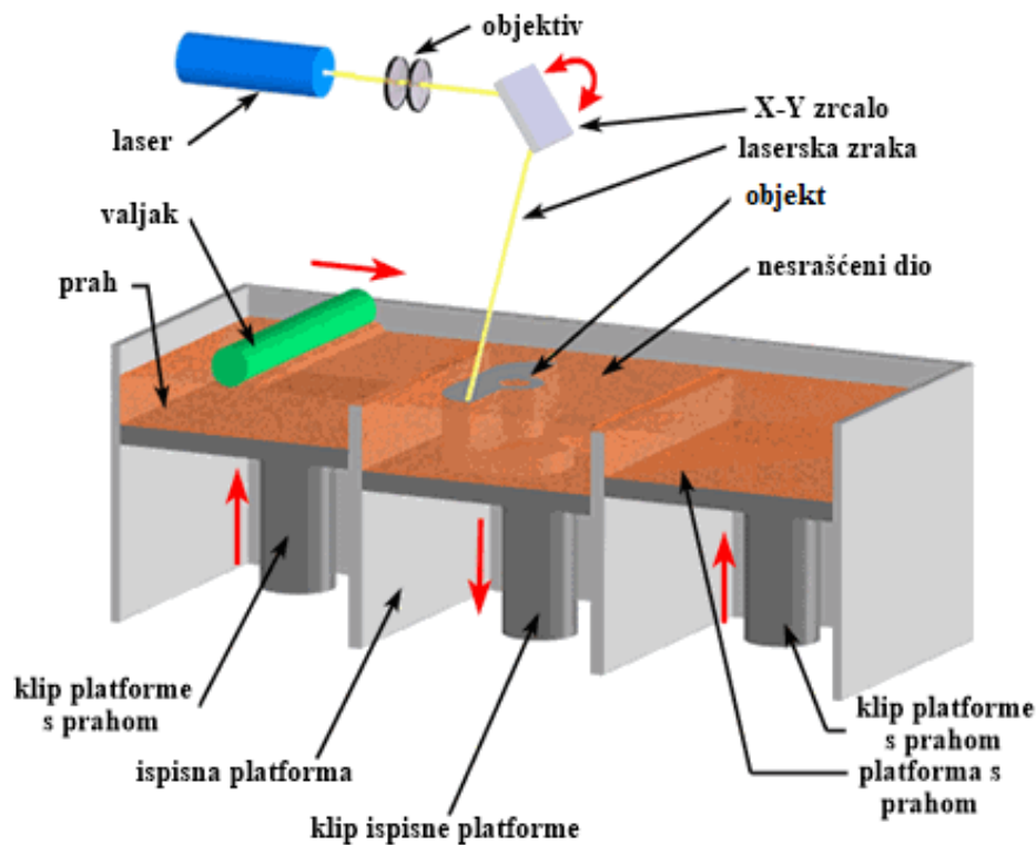
Slika 3.1. Selektivno lasersko sraščivanje [20]
