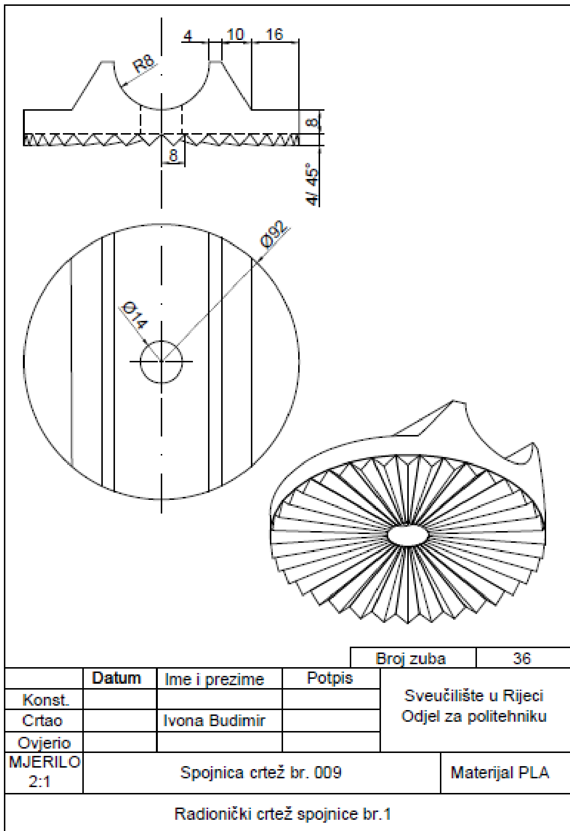
Slika 5.2. Radionički crtež spojnice br.1
