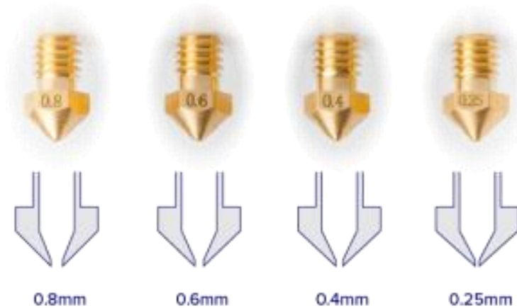
Slika 4.6. Debljine mlaznica [39]
