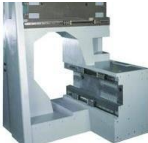
Slika 4.1. Konstrukcija stroja od polimernog betona
