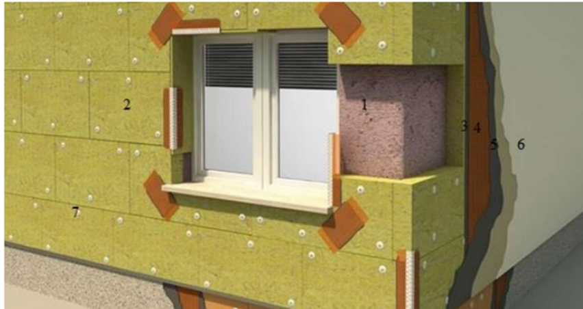
Slika 8. Zvučna i toplinska izolacija vanjskog zida građevine. Nosivi zid (1), ploča od kamena (2), Građevinsko ljepilo (3), Mrežica (4), Građevinsko ljepilo(5), Završni sloj(6), Tiple (7), Zona prskanja izoliranim ekstrudiranim polistirenom (8) (DELTAPLUS, 2020)
