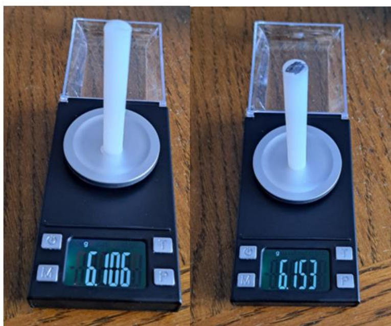
Slika 7 Rezultati mjerenja poliamida PA 6 prvog dana
