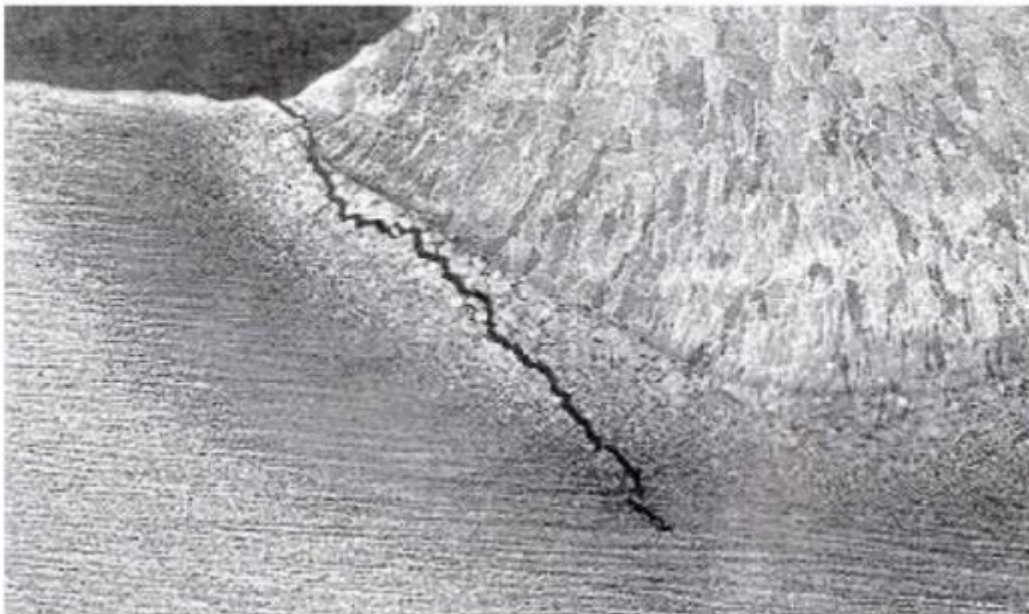
Slika 3.3. Nastajanje hladne pukotine [6]
